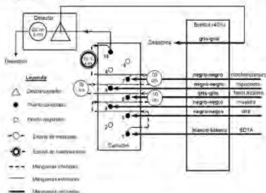
Fig. B.7.4-2. Configuración del cartucho para el análisis de \text{N-NH}_4 .
