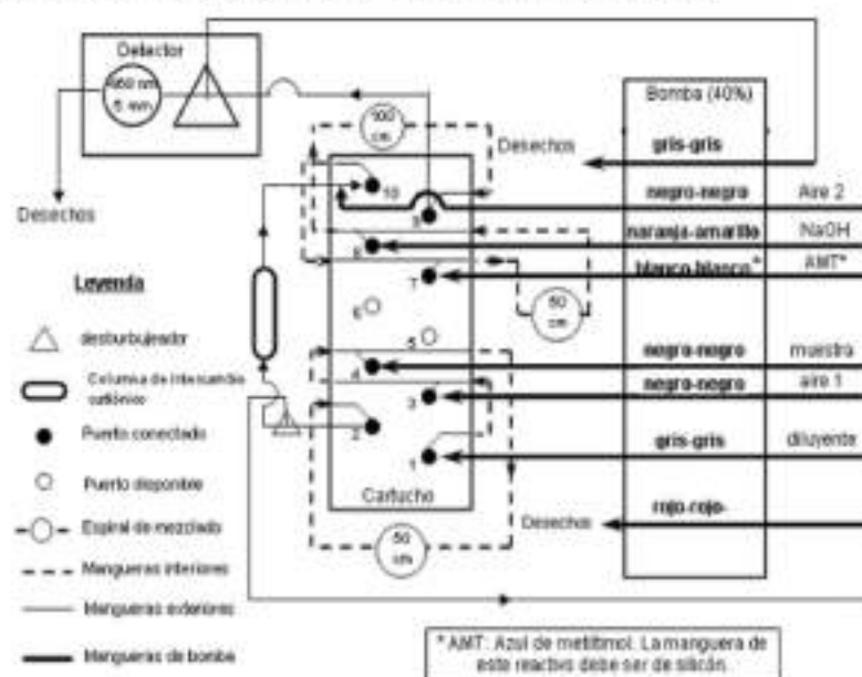
Fig. B.11.2-2. Configuración del cartucho para el análisis de sulfato en el intervalo de 5.0-200 mg/L.
