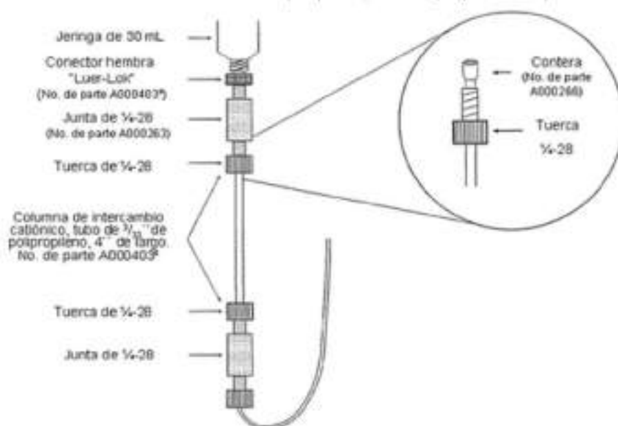
Figura B.11.2-3. Partes de la columna de intercambio catiónico.
