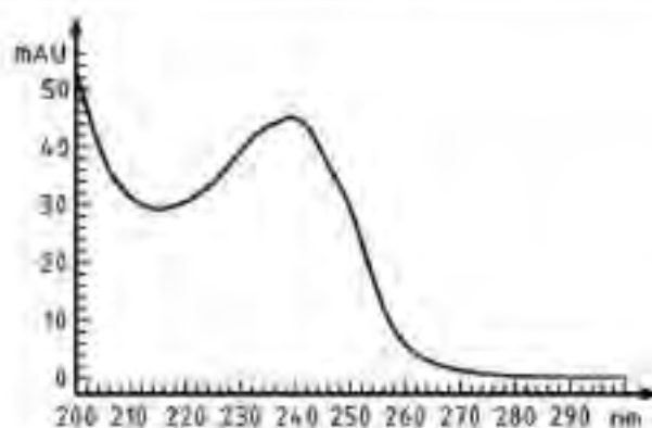
c) Espectro de absorción típico de MC-LR en un sistema de acetónitrilo/agua
