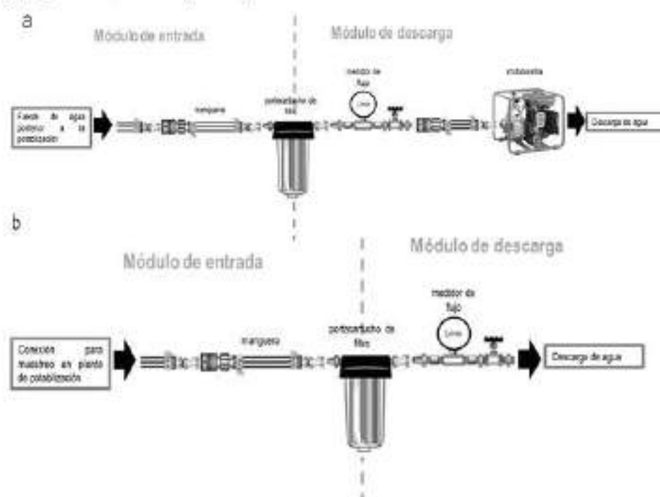
Fig. B.2.1.1 Dispositivo de muestreo. 1a) en caso de existir conexión para muestreo a la salida de la planta de potabilización. 1b) en caso de no existir conexión para muestreo a la salida de la planta de potabilización.
