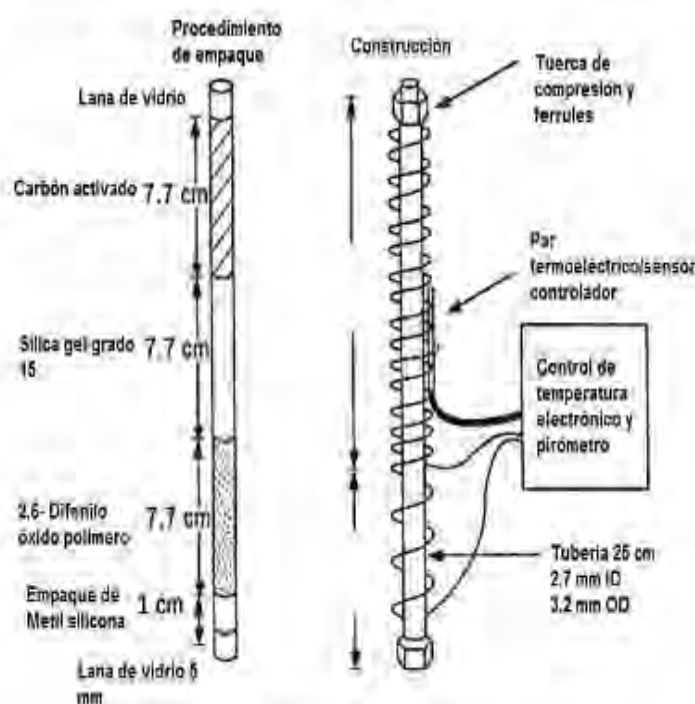
Fig. B.3-2. Especificaciones del ejemplo de trampa
