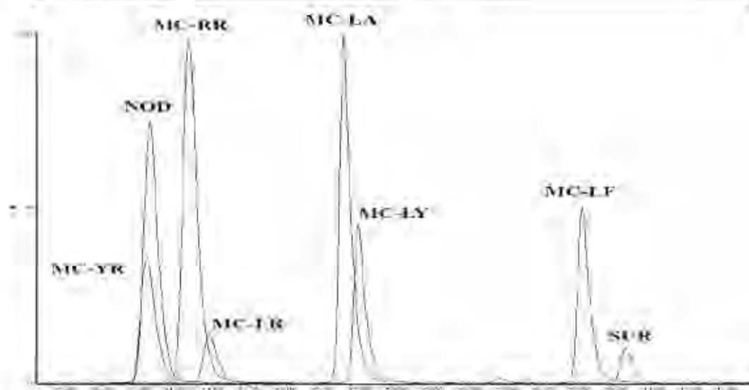
Fig. B.1.2.2 Ejemplo de cromatograma (segmentos MS/MS sobrelapados) de un estándar de calibración con el método 544 de EPA y con analitos en una concentración de 187.5-1 000 ng/L.
