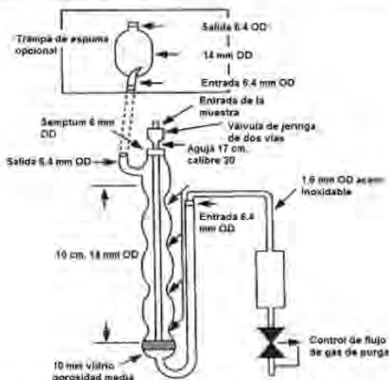
Fig. B.3-1 Dispositivo de purga. Se incluye sólo como ejemplo y no implican aprobación de los productos. Pretende únicamente representar especificaciones adecuadas para los artículos.
