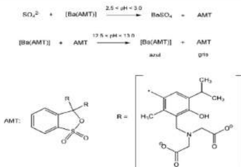
Fig. B.11.2-1. Reacción entre el ion sulfato y el complejo bario – azul de metiltilmol (Ba-AMT).
