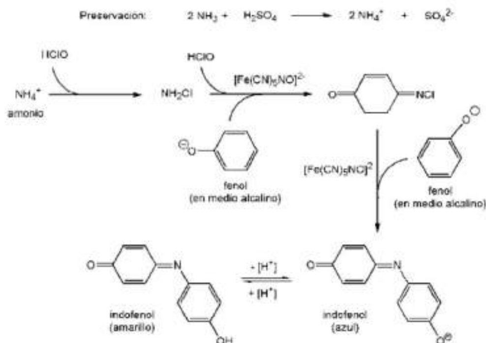
Fig. B.7.4-1. Formación del indofenol de color azul producto de la reacción del ión amonio con hipoclorito y fenol en medio básico en presencia de nitroferrocianuro.
